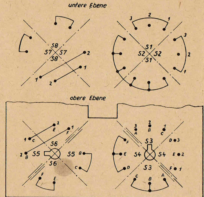
'Schalteransichten von hinten auf die Ebenen gesehen'
